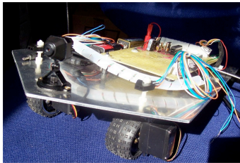
Tripè: robot a ruote supleconomico
